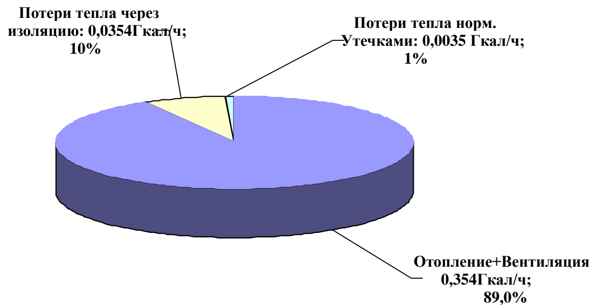
Рис.1.3.Соотношение нагрузок отопления, вентиляции и расчетных потерь в системах теплоснабжения Ровеньского района от всех источников теплоты
