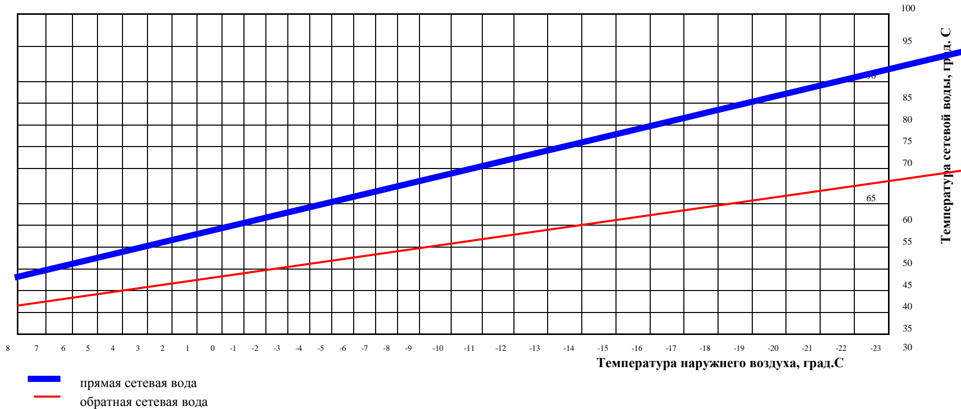
Рис.5.1. Расчетный температурный график регулирования отпуска тепловой энергии от котельной с.Айдар и с.Пристень
